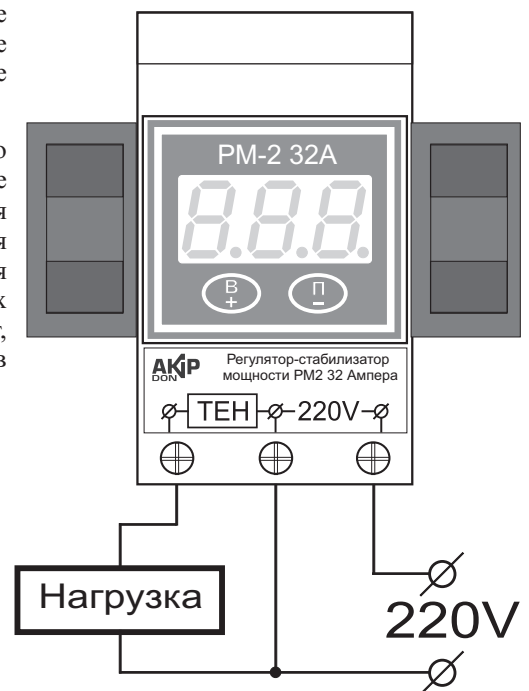
Рис. 1. Схема монтажа прибора.
