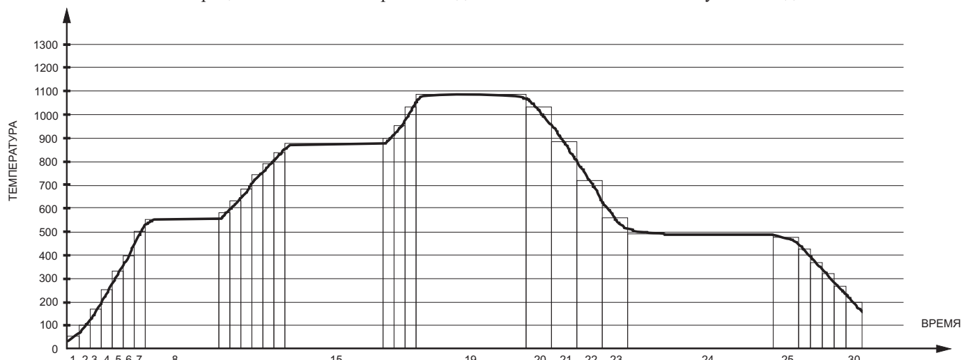
Рис.2 Условная схема профиля техпроцесса на 30 заданий (позиций) температура-время.
