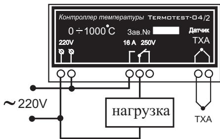
Рис.2 Схема подключения.
