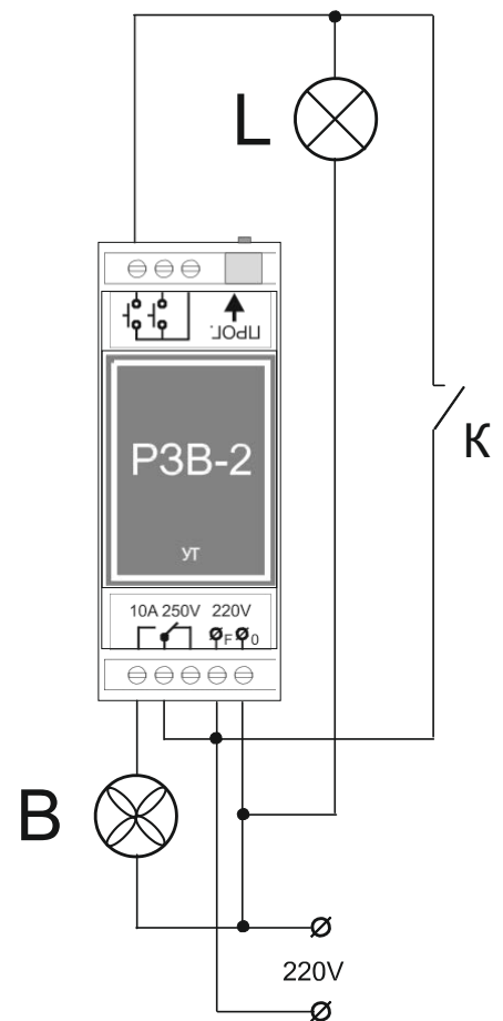
Рис 3. При замыкании контакта К лампа Л и вентилятор В включается, после размыкания лампа выключается и начинается отсчет времени по истечении которого выключается вентилятор. В качестве К применяется обычный выключатель.
