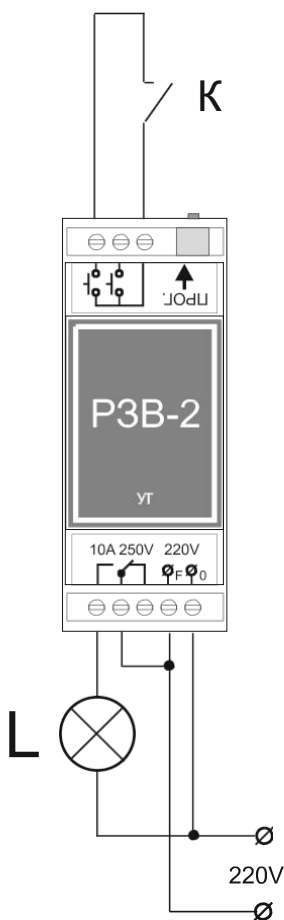
Рис 1. При замыкании контакта К лампа Л включается, после размыкания начинается отсчет времени по истечении которого лампа выключается. В качестве К может быть кнопка без фиксации или обычный выключатель.
