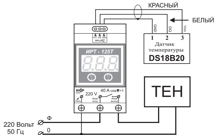
Рис. 2. Схема монтажа прибора с 3х проводным подключением датчика.
